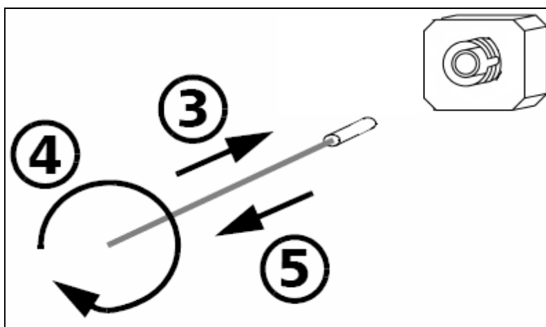
Рис. 40 Чистка разъемов
