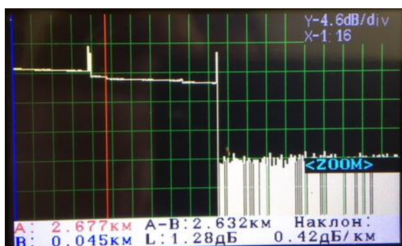
Рис. 14. Изменение масштаба рефлектограммы.
