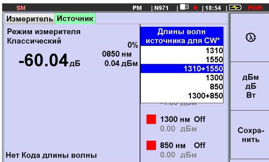
Рис.6.8.. Длины волн в режиме излучения источника CW*.
