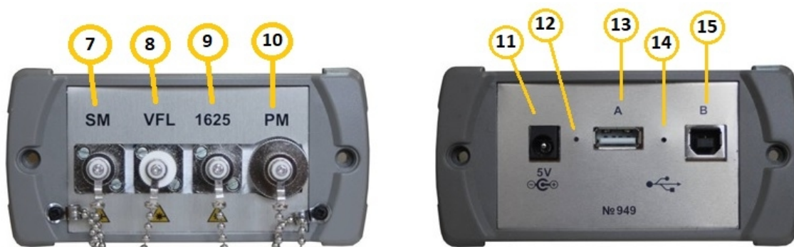
Рис.4.2. Виды слева (оптические разъемы) и справа (электрические разъемы)
