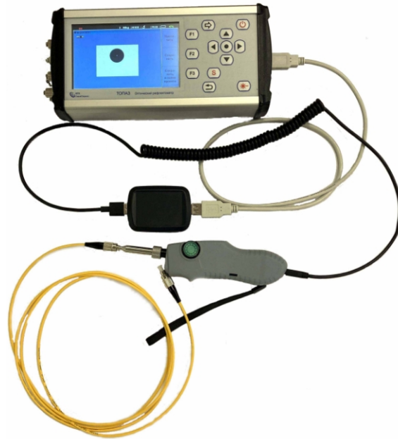
Рис.7.2. Подключение Волоконного микроскопа к рефлектометру «Топаз-9400»
