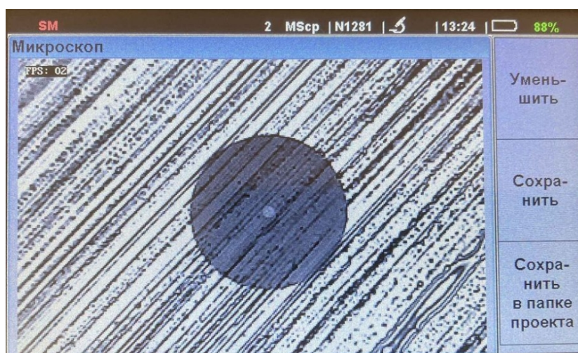
Рис. 7.6. Изображение поверхности тестируемого коннектора после нажатия «F1»
