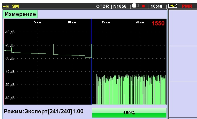
Рис. 5.16. Процесс измерения
